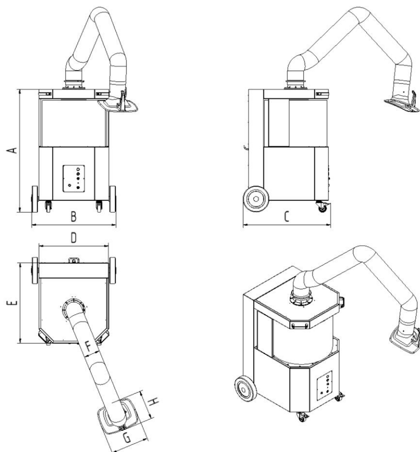
Fig. 7: Disegno quotato
