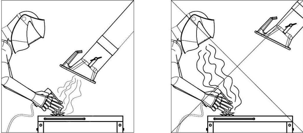
Fig. 4: Posizionamento della cappa di aspirazione
