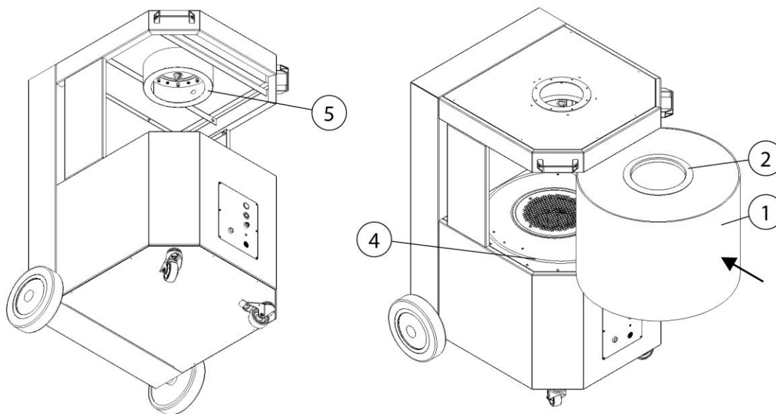
Fig. 6: Cambio filtro - Inserire l'elemento filtrante
